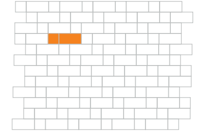
Брусчатка 200x100x60 мм Декор 100x100x60 мм
