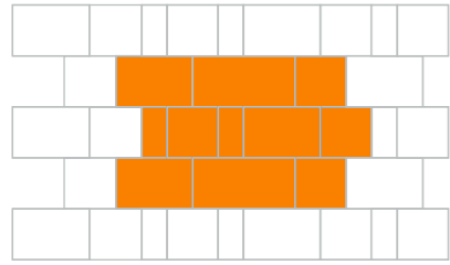
Урбан 498x248x80 мм 373x248x80 мм 248x248x80 мм 123x248x80 мм
