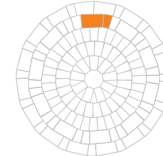
Трапеция 95,8x121x60 мм 175,8x121x60 мм
